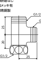
分岐継手 PZ438KN ¥1,700(税込¥1,870) [1-] ■研磨なし ■メッキ有 ■青銅製
