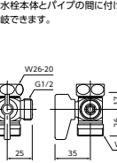
切替ボール弁 ZK73 ¥3,870(税込¥4,257) [5-] ■水栓本体とパイプの間に付けて分岐できます。
