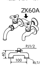
二又ソケット13(1/2)用 ZK60A ¥3,510(税込¥3,861) [4-] ■1つの配管に水栓を2つ付ける
