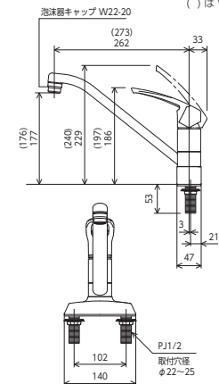
KM5081T(V8)
