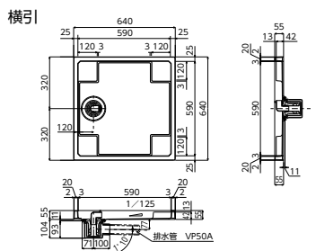
洗濯機パン VR26-PTN トラップなし ¥13,860 (税込¥15,246) [5] ■排水トラップは別売です。 ■耐荷重200kg
