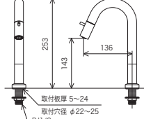
K1103L2 <取付工具 KPS953 >
