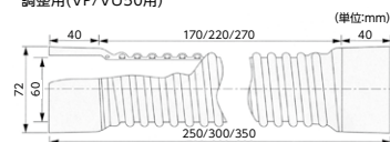
フレキシブルジョイント(洗濯機パン接続用) ZY15-250 *規定在庫品 250mm ¥3,390 (税込¥3,729) [120]
