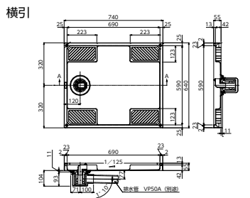
洗濯機パン(ドラム式対応) VR30-PTN トラップなし ¥15,620 (税込¥17,182) [5] ■排水トラップは別売です。 ■耐荷重200kg
