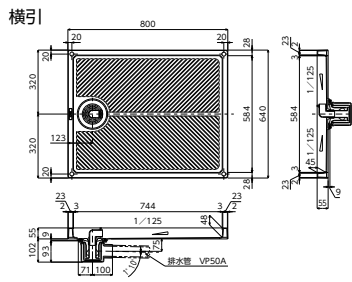
洗濯機パン VR21-PTN トラップなし ¥16,280 (税込¥17,908) [5] ■排水トラップは別売です。 ■耐荷重200kg
