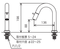
K1103L <取付工具 KPS953 >
