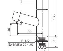
K550 <取付工具 G4 >
