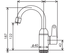
K103GT <取付工具 G4 >
