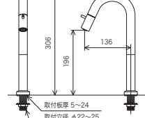
K1103L3 <取付工具 KPS953 >
