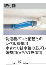
取付例 ・洗濯機パンと配管とのレベル調整用 ・水まわり排水管の芯ズレ調整用(VP/VU50用)
