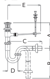
寸法図
