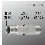
ステンレスニップル ■-の後ろの数字は長さ(mm) ※Z698-75のみ表面に光沢があります。
