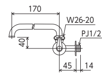
横形自在水栓 K10E [1/20] ¥6,300 (税込¥6,930) JIS プチ エコ こま ■固定こま ■節水チップ内蔵型
