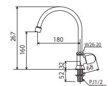
泡沫立形自在水栓 K16NDSFFER2 [1/10] ¥9,430 (税込¥10,373) JIS 泡沫 プチ エコ こま ■固定こま ■節水チップ内蔵型
