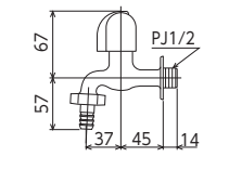
カップリング付横水栓 K4EJ [1/40] ¥6,400 (税込¥7,040) K4EZ [1/40] 逆止弁 エコ こま ¥5,700 (税込¥6,270) JIS 逆止弁 エコ こま ■固定こま ■節水チップ内蔵型 ■寒冷地用は逆止弁なし
