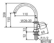
立形自在水栓 K16NDSSE [1/20] ¥7,250 (税込¥7,975) JIS プチ エコ こま ■固定こま ■節水チップ内蔵型
