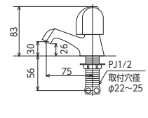
立水栓 K5E [1/40] ¥6,900 (税込¥7,590) JIS プチ エコ こま 部品一覧P.450 ■固定こま ■節水チップ内蔵型
