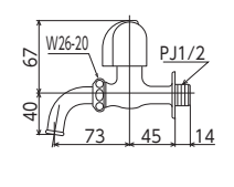
吐水口回転形水栓 K11E [1/40] ¥5,300 (税込¥5,830) JIS プチ エコ こま 部品一覧P.453 ■固定こま ■節水チップ内蔵型
