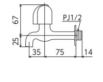
胴長横水栓 K2E [1/40] ¥5,800 (税込¥6,380) JIS プチ エコ こま ■固定こま ■節水チップ内蔵型
