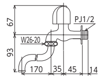
自在水栓 K3E [1/20] ¥6,000 (税込¥6,600) JIS プチ エコ こま ■固定こま ■節水チップ内蔵型
