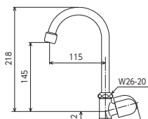
泡沫立形自在水栓 K16NDSFFC [1/20] ¥8,800 (税込¥9,680) JIS 泡沫 プチ エコ こま ■固定こま ■節水チップ内蔵型
