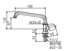
立形自在水栓 K16NDE [1/20] ¥6,650 (税込¥7,315) JIS プチ エコ こま ■固定こま ■節水チップ内蔵型
