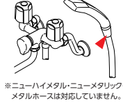
シャワーホースナットセット PZKF171S ¥1,550(税込¥1,705) [10] ■シャワーヘッド側φ16用 ■M22×2
