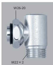
流量調節付シャワーエルボ 袋ナット接続タイプ Z416660 ¥4,050(税込¥4,455) [1] ■W26-20・M22×2 ※シャワーホース接続用です。
