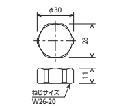
キャップナット Z750 ¥890(税込¥979) [1] ■樹脂製 ■W26-20
