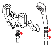
シャワーホースパッキンセット PZKF26-3 ¥340(税込¥374) [10] ※ニューハイメタルホース・ニューメタリックホースは対応していません。
