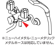
シャワーホース六角ナットセット PZKF172S ¥1,190(税込¥1,309) [10] ■シャワー本体側φ16用 ■M22×2
