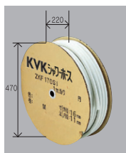
シャワーホース ZKF170SSI-25 25m ¥22,000(税込¥24,200) [1] ZKF170SSI-50 50m ¥38,280(税込¥42,108) [1] ZKF170SSI-100 100m ¥69,410(税込¥76,351) [1] ■外径16×内径11mm ■白ホース
