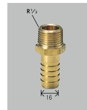
ホースニップル13(1/2)x16φ用 Z1018 ¥680 (税込¥748) [40] [20]
