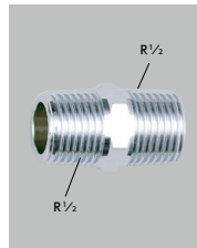
ニップル13(1/2)用 Z737-13 ¥410 (税込¥451) [25] [20]
