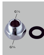
20(めねじ)x13(おねじ)アダプター Z187 ¥810 (税込¥891) [10] [20]
