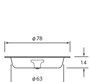
流し排水栓目皿 PZ1033 ¥700(税込¥770) [10]
