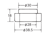
排水ホースキャップ PZ1039 ¥320(税込¥352) [20]
