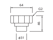
排水ホースユニオンナット PZ1037-2 ¥740(税込¥814) [10]
