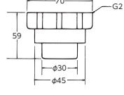
排水ホースナット PZ1040-2 ¥650(税込¥715) [10]
