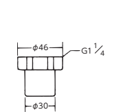
排水ホースユニオンナット PZ26 ¥590(税込¥649) [10]
