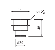
排水ホースユニオンナット PZ1037-1 ¥570(税込¥627) [10]
