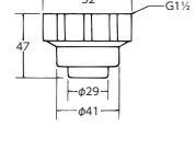
排水ホースナット PZ1040 ¥570(税込¥627) [10]
